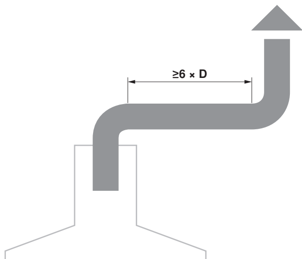
Tracciato dei tubi ideale
