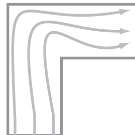
Andamenti squadrati e spigolosi devono essere evitati.
