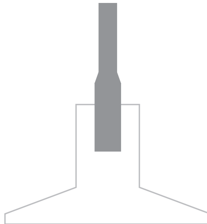
Restringimento della sezione trasversale
