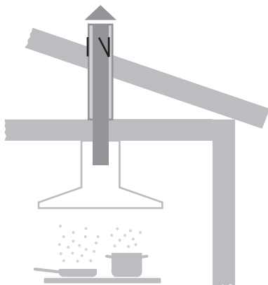
Con sbocco nel tetto
