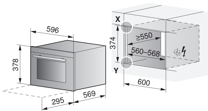
Frontmasse der Geräte: Detail X/Y (siehe Seite 12)
