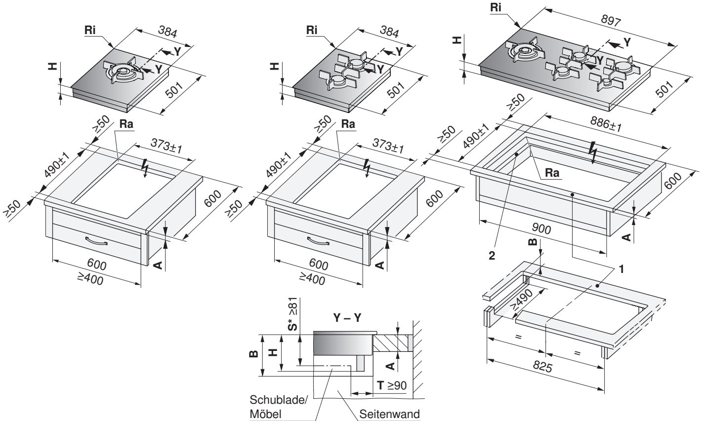
GAS411GSAZ/GSBZ (31063)
