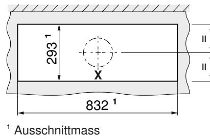
Ausschnitt Oberschrank (Ansicht X)
