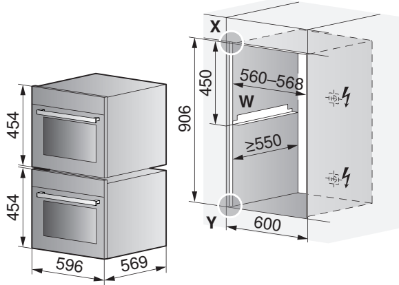
Frontmasse der Geräte: Detail X/Y (siehe Seite 12)
