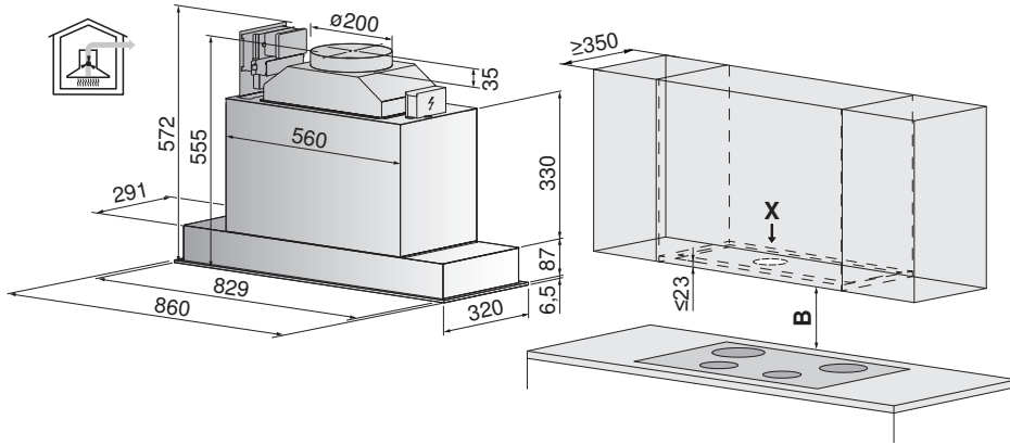
Ausschnitt Oberschrank (Ansicht X)
