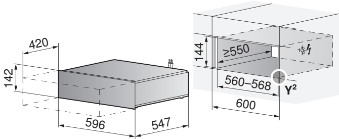
WS60144 (34017) Einzeleinbau
