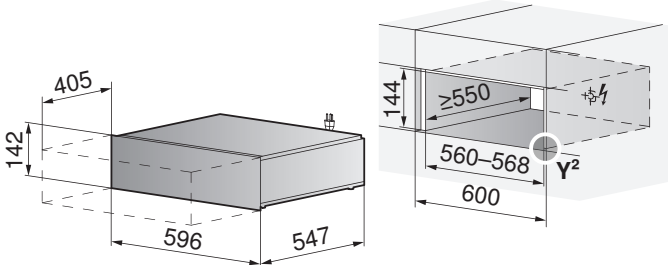
VS60144 (36001) Einzeleinbau
