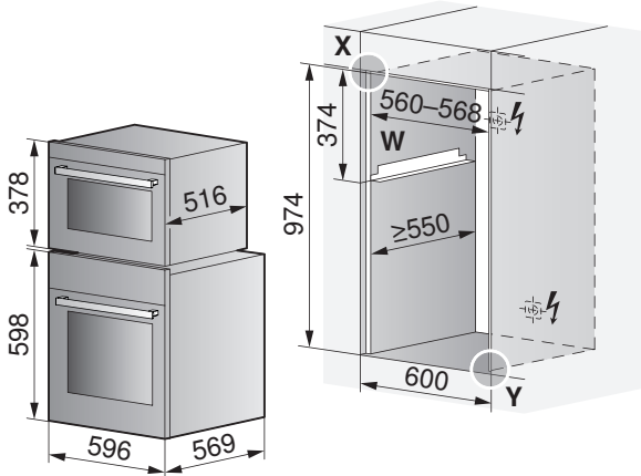
Frontmasse der Geräte: Detail X/Y (siehe Seite 12)
