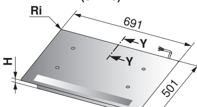
CookTopInduktion V4000 (31116)
