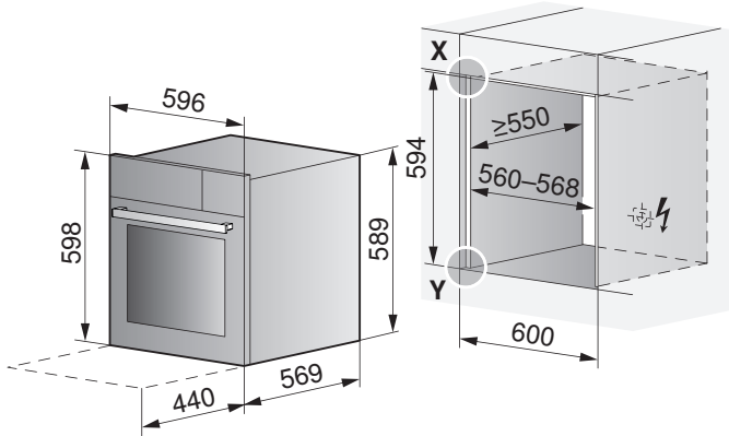
Frontmasse der Geräte: Detail X/Y (siehe Seite 12)
