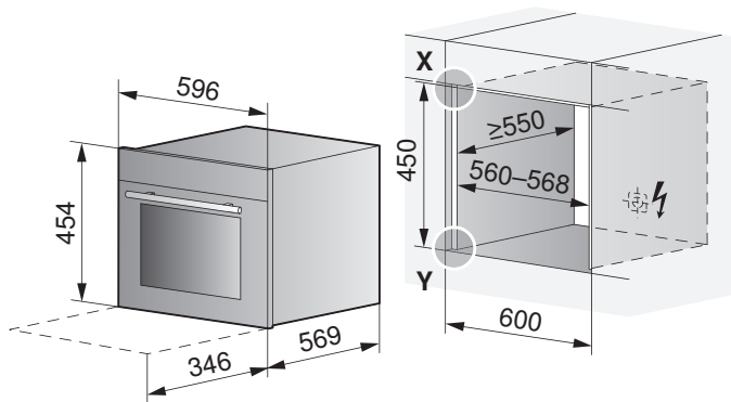
Frontmasse der Geräte: Detail X/Y (siehe Seite 12)
