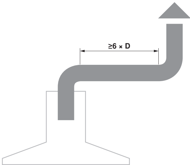
Guter Rohrverlauf
