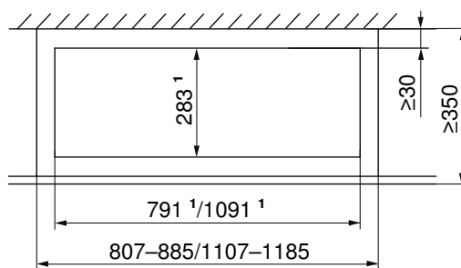
Découpe armoire suspendue (vue X)
