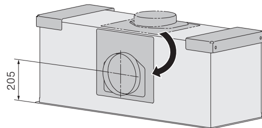
Vue Y
